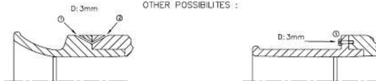
TEKENING 254-4
