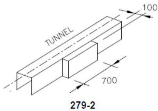
Afbeelding-279-2
