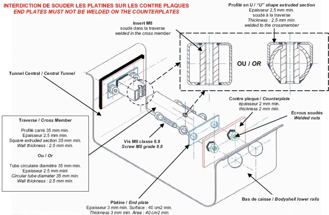
Tekening 253-65B
