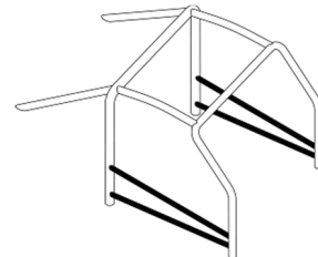
Tekening 253-11
