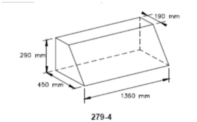
Afbeelding-279-4
